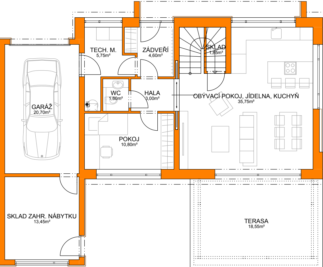
Půdorys 1.NP
