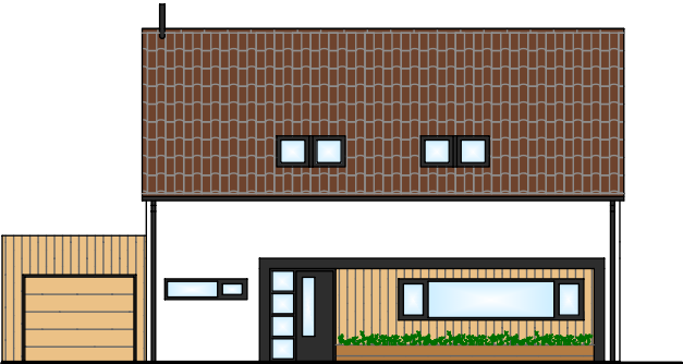
POHLED OD JIHU - ULIČNÍ
