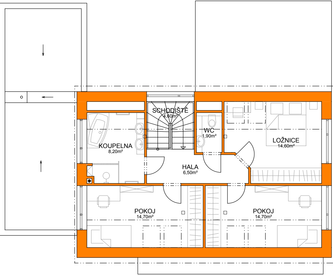
Půdorys 2.NP
