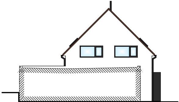
POHLED OD ZÁPADU
