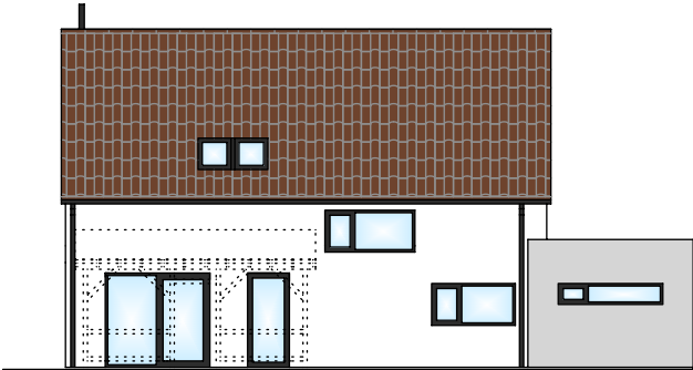
POHLED OD SEVERU
