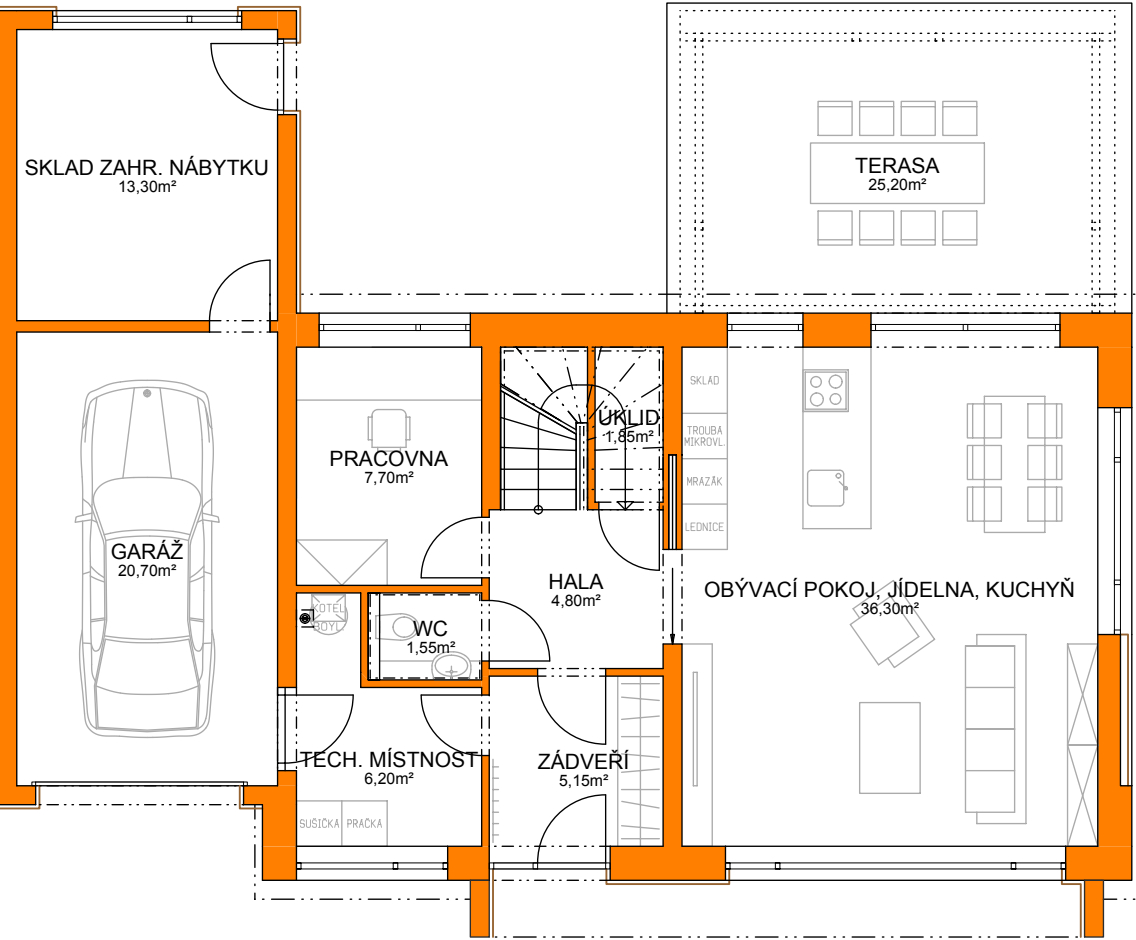
Půdorys 1.NP
