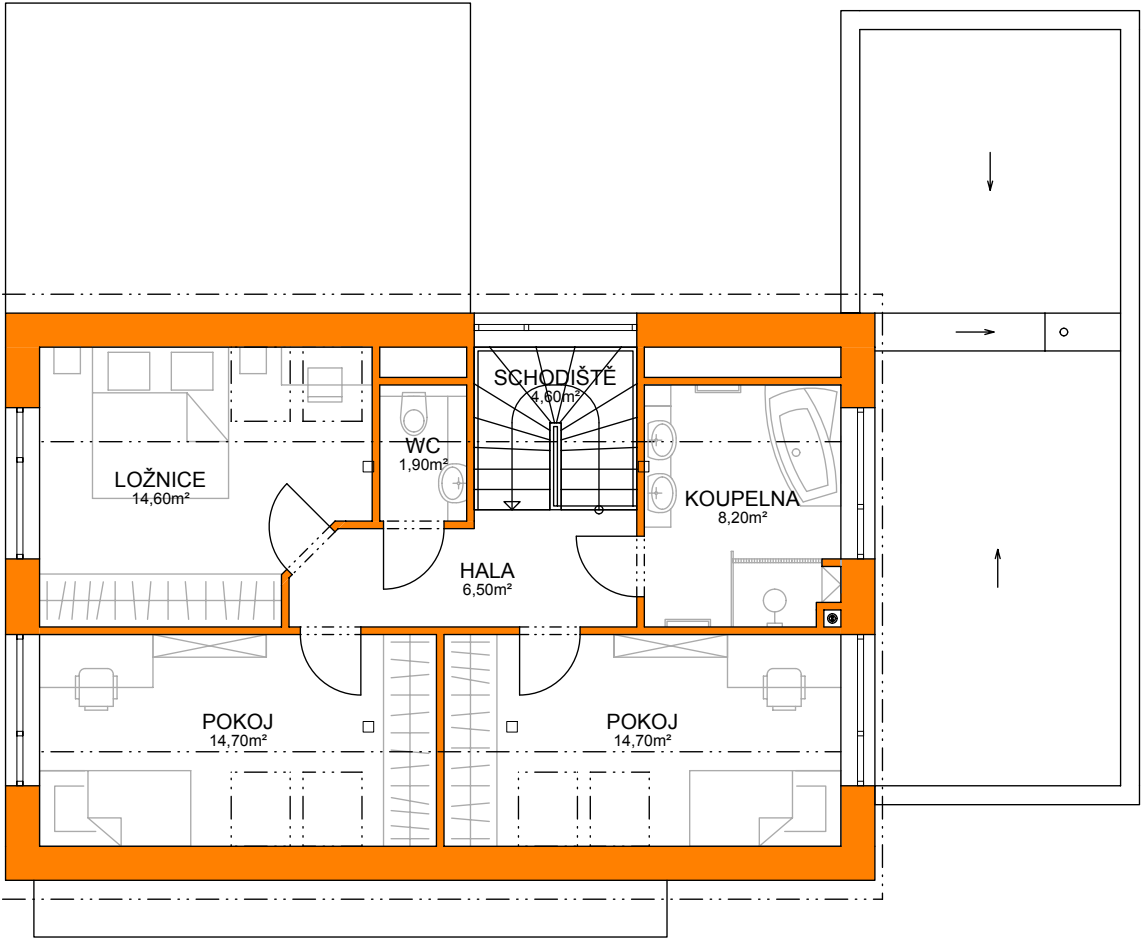
Půdorys 2.NP
