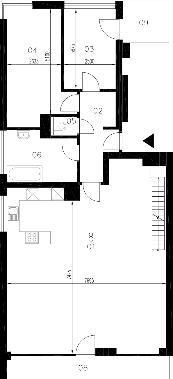
3. NADZEMNÍ PODLAŽÍ BYT 8 3+KK
