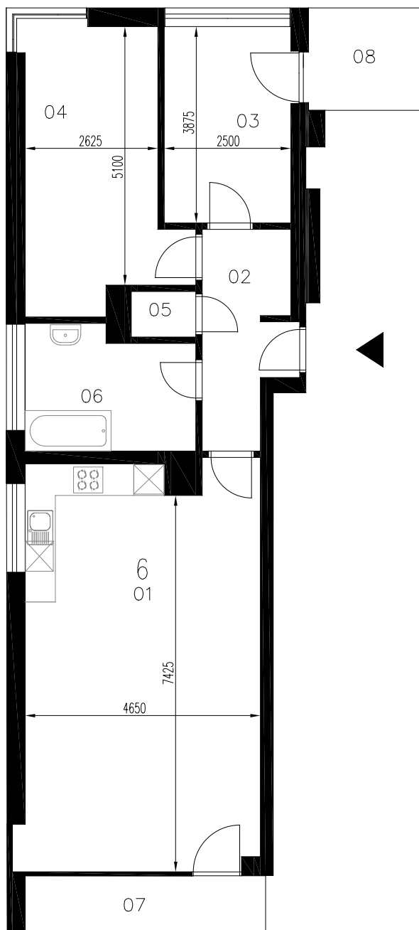
2. NADZEMNÍ PODLAŽÍ BYT 6 3+KK
